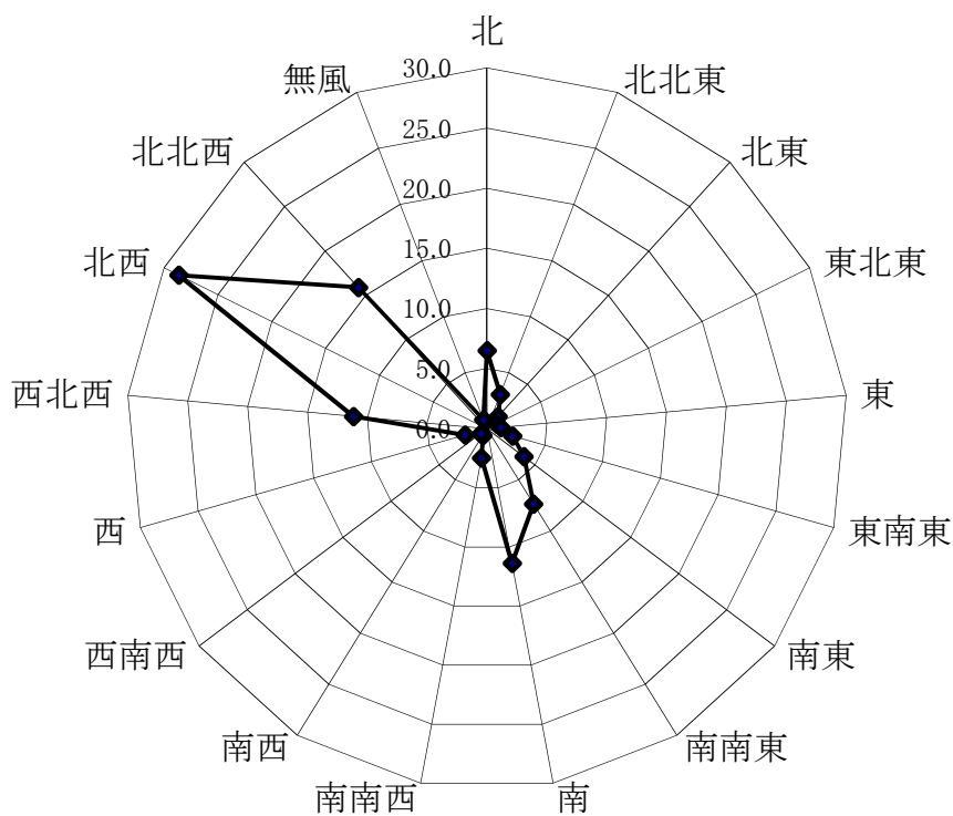
年間風向状況(%)
