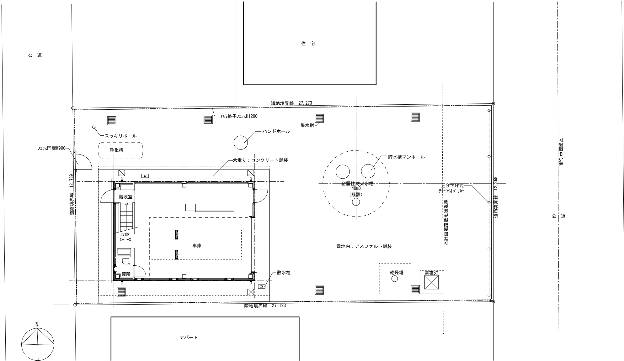
配置図・1F平面図 1/100
