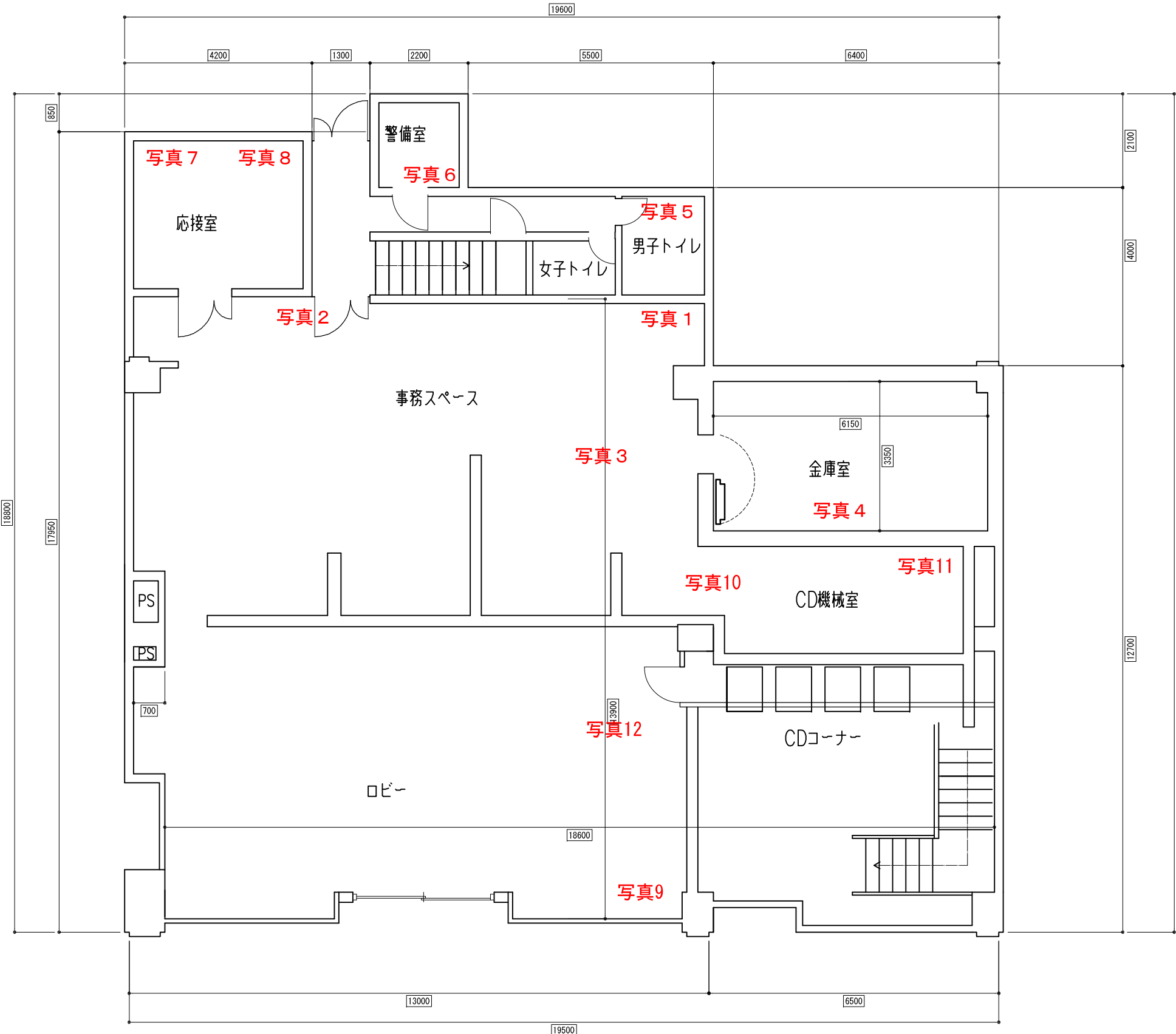
1階 平面図
